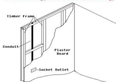
Conduit Wiring (concealed conduit wiring)
